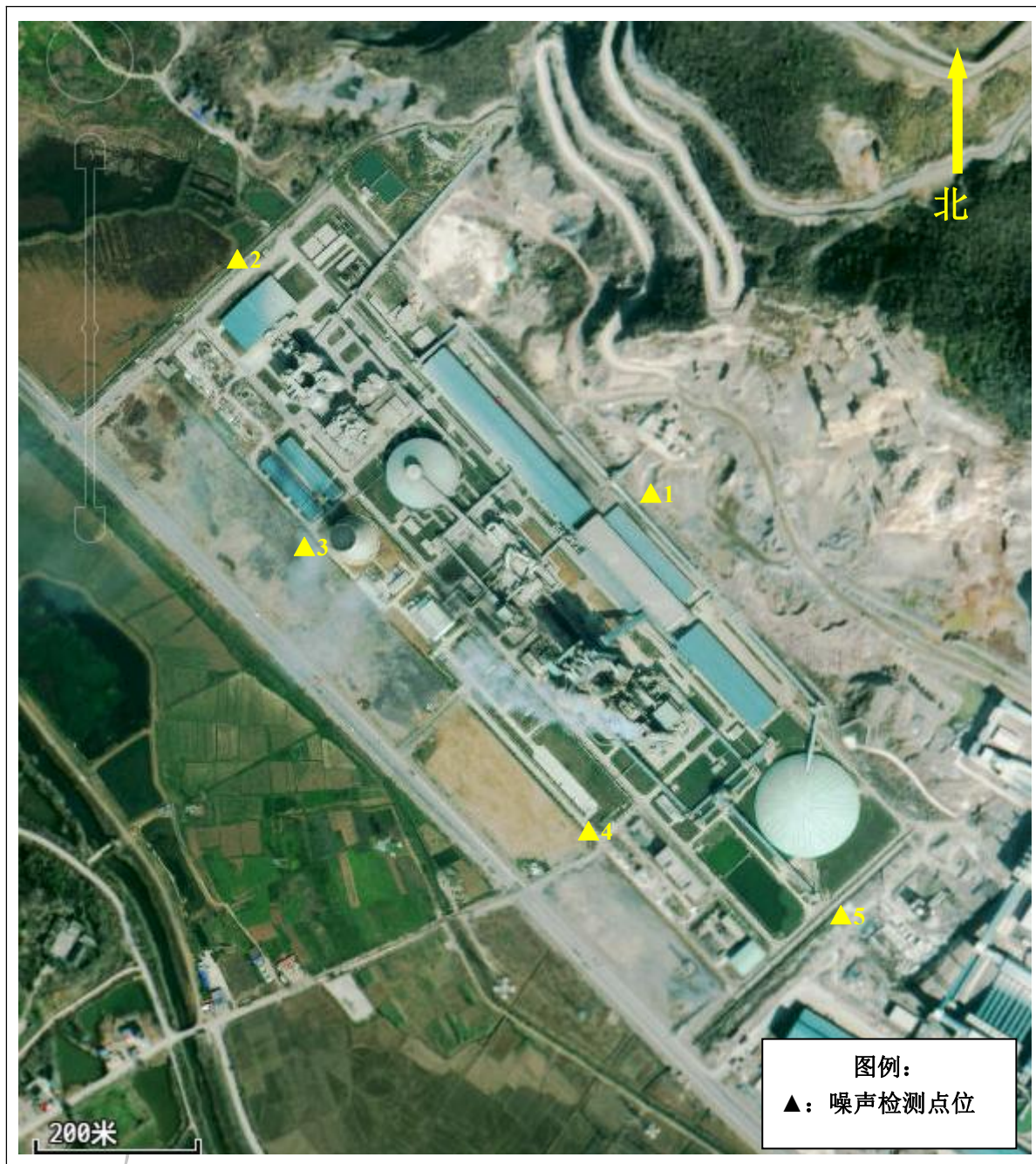
附图 1：现场检测点位平面布置图
